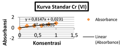
Gambar 4.1 Kurva standar Cr(VI)
