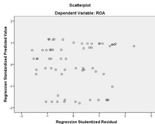
Gambar 4.1 Hasil Uji Heterokedastisitas
