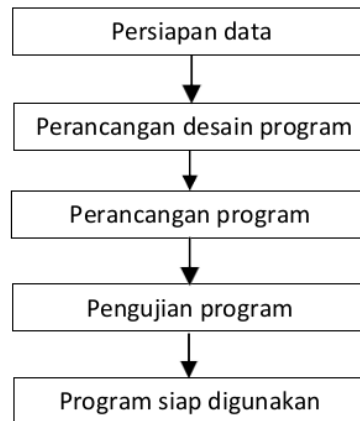
Gambar 2. Metodologi penelitian
