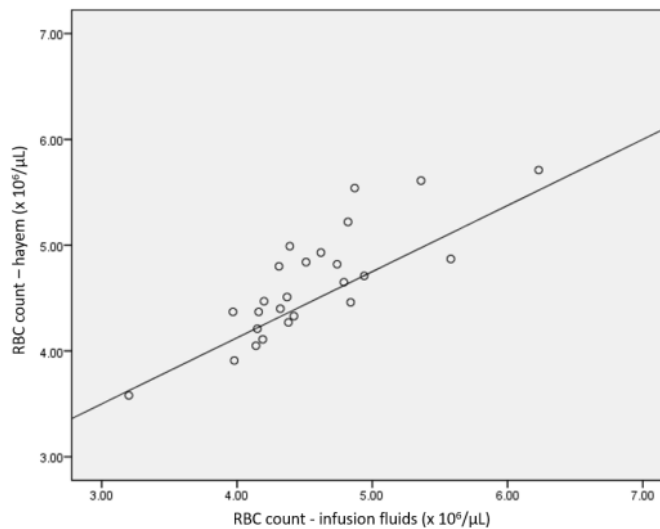
Gambar 2. Grafik uji regresi linier pemeriksaan RBC cairan infus 0,9% terhadap pemeriksaan RBC reagen Hayem.
