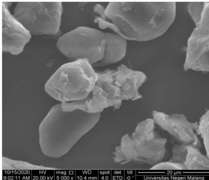
Gambar 4. Morfologi nanopartikel As-CP-NP-BSA dengan SEM-EDX
