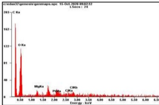
Gambar 5. Unsur dan Komposisi Unsur Hasil Analisis SEM-EDX
