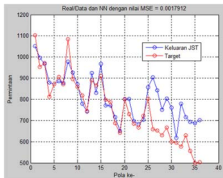
Gambar 2 Hasil pelatihan WB epoch 3000
