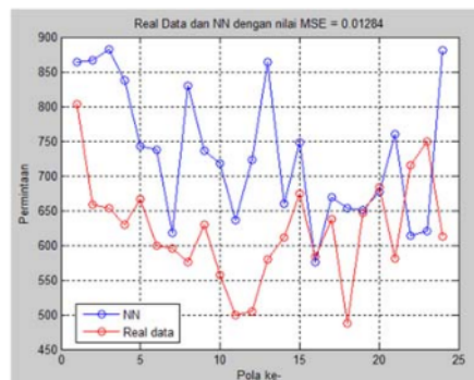
Gambar 6 Hasil pengujian WB epoch 4000
