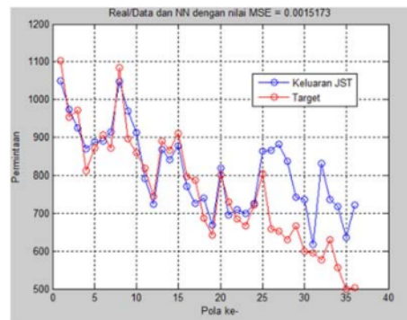
Gambar 3 Hasil pelatihan WB epoch 4000
