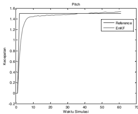
Gambar 4. Estimasi gerak Pitch dengan membangkitkan 300 Ensemble
