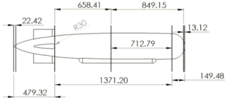
Gambar 1. Profil dari ITSUNUSA AUV (Teguh Herlambang & Subchan, 2018)
