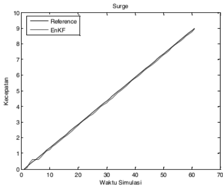
Gambar 2. Estimasi gerak dengan membangkitkan 200 Ensemble
