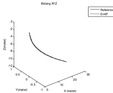
Gambar 5. Estimasi Lintasan Menyelam dengan membangkitkan 300 Ensemble
