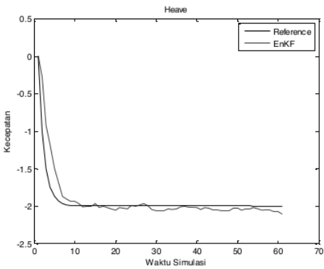
Gambar 3. Estimasi gerak Heave dengan membangkitkan 300 Ensemble
