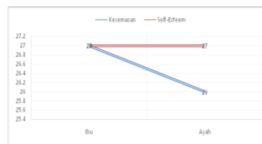
Grafik 3. Nilai Rata-rata Hubungan Antara Gaya Pengasuhan Ibu dan Ayah
