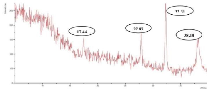
Gambar 4. Hasil Spektrum Pola Difraksi XRD
