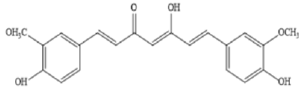
Gambar 1. Struktur Kurkumin. Sumber (Naama, Al-temimi, et al., 2010)
