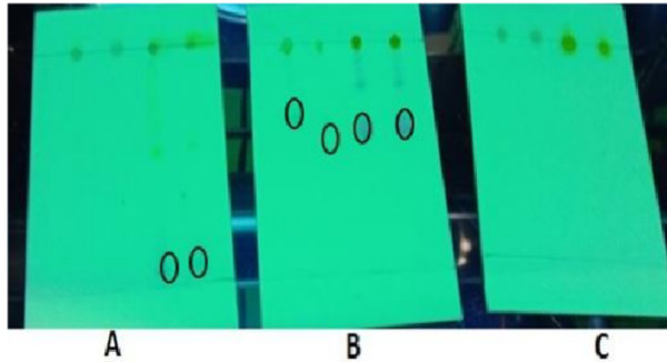
Gambar 3. Hasil analisis KLT (a) Kloroform: Etanol, 2 Noda, (b) Kloroform: Heksana, 4 Noda, (c) Kloroform: Benzena: Metanol, 0 Noda
